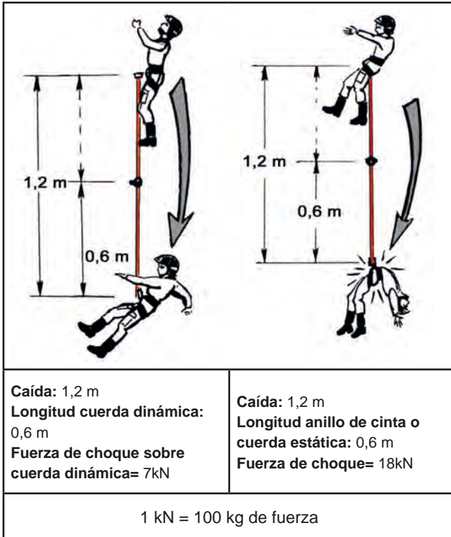
Imagen 10. Fuerza de choque según tipo de cuerda
