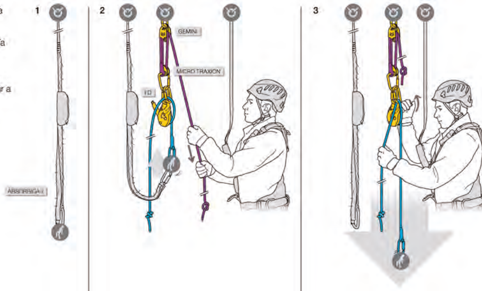
Imagen 95. Evacuación sin acompañamiento
