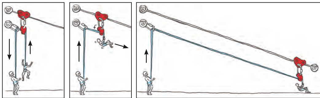
Imagen 103. Uso del polipasto para salvar obstáculos
