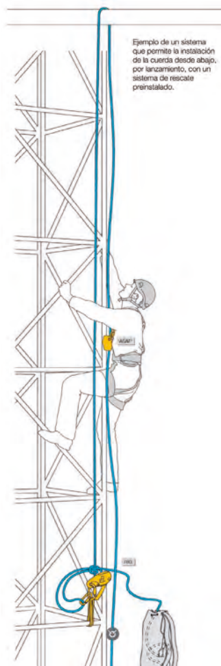
Imagen 63. Ascenso asegurado con anticaidas
