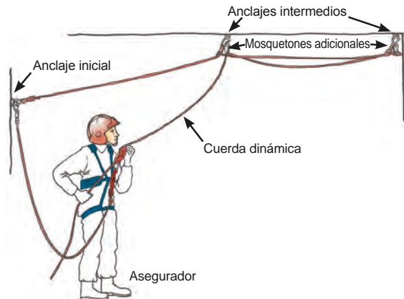
Imagen 66. Montaje de línea de vida horizontal provisional
