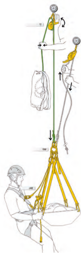
Imagen 93. Cuerda anclada en “V”
