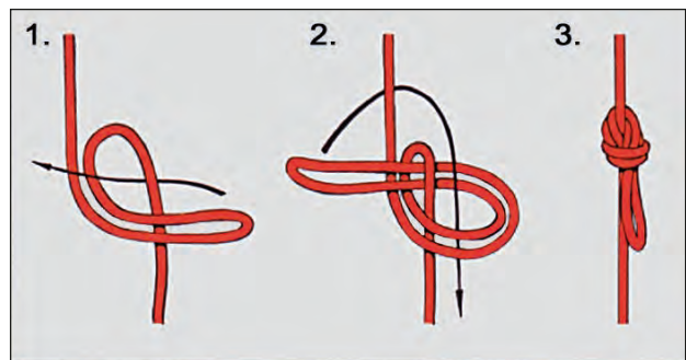
Imagen 38. Nudos direccionales. Nudo romano
